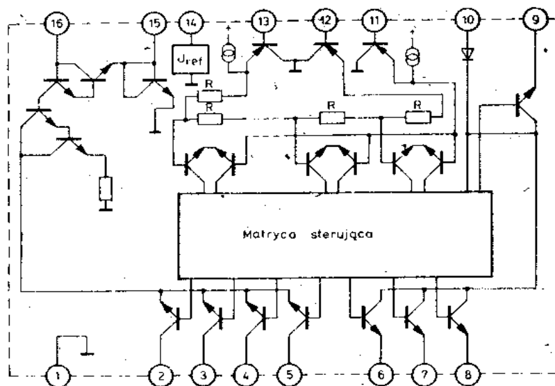
Schemat blokowy
