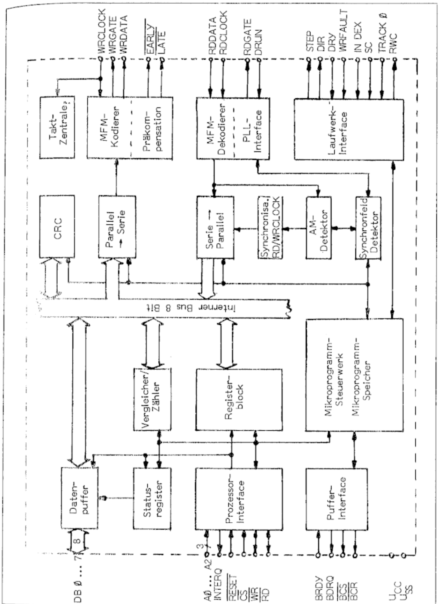
Übersichtsschaltplan
