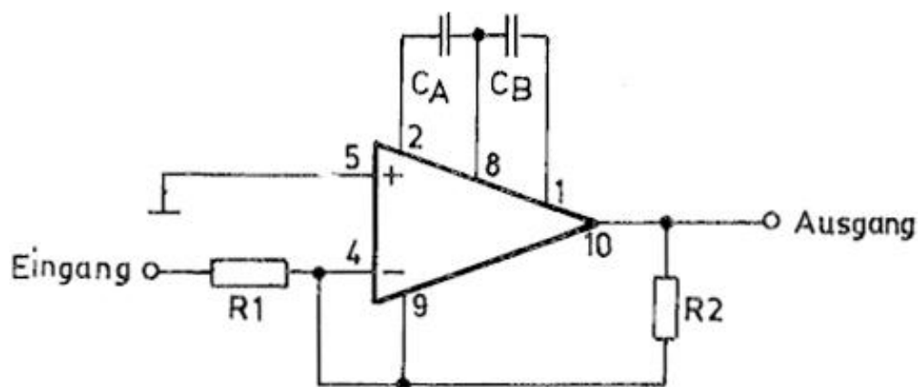
Applikationsschaltung: nichtinvertierender Verstärker
