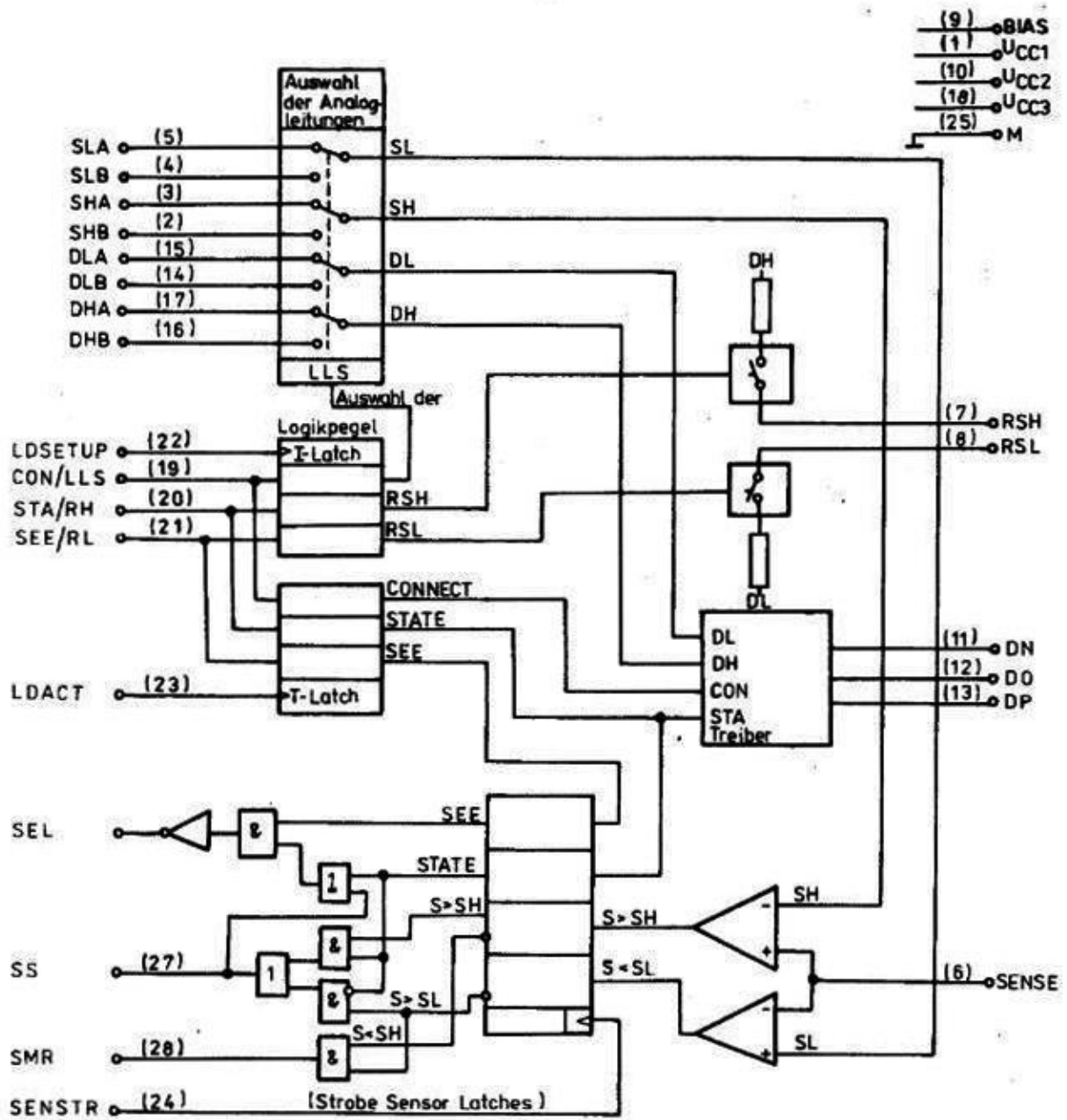
Bild 3: Blockschaltbild
