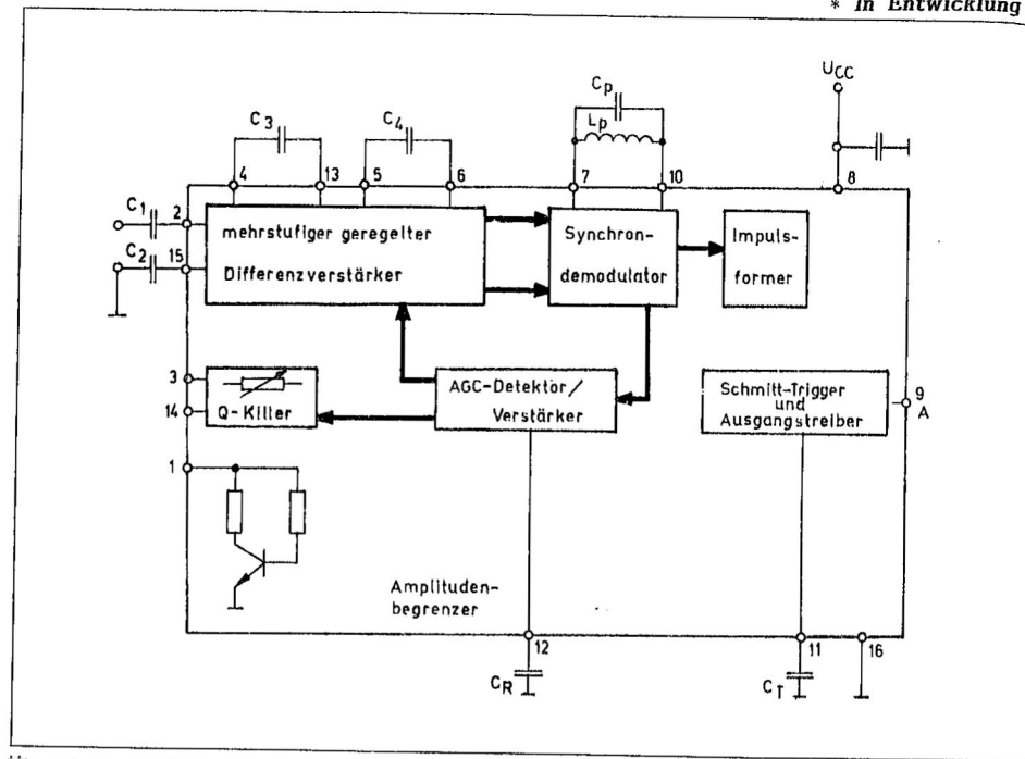
Übersichtsschaltplan
